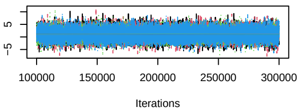
Trace of d.Erlotinib.Erlotinib_IGF_1Ri
