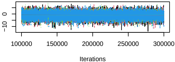
Trace of d.Erlotinib.Erlotinib_chemo
