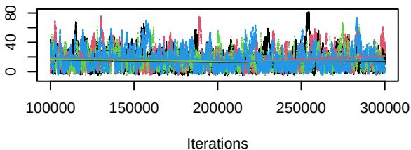
Trace of d.Erlotinib.Erlotinib_HER3i
