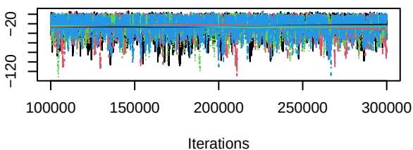
Trace of d.Erlotinib.Erlotinib_HGFi
