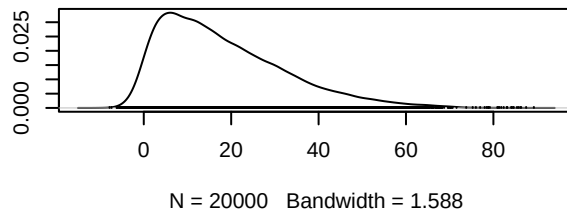
Density of d.Gefitinib.Gefitinib_PARPi
