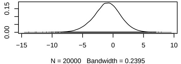
Density of d.Erlotinib.Erlotinib_chemo
